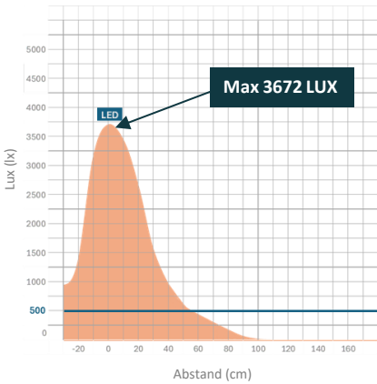
Lux-Messung der Beleuchtungsstärke aus der Seitenansicht in 40 cm Abstand
