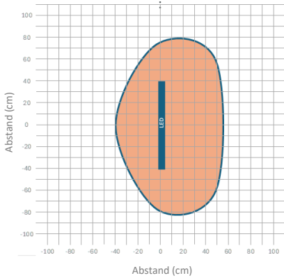
Lux-Messung der Beleuchtungsstärke aus der Draufsicht in 40 cm Abstand
