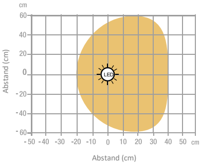
Lux-Messung der Beleuchtungsstärke aus der Draufsicht in 40 cm Abstand
