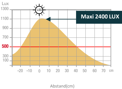
Lux-Messung der Beleuchtungsstärke aus der Seitenansicht in 40 cm Abstand
